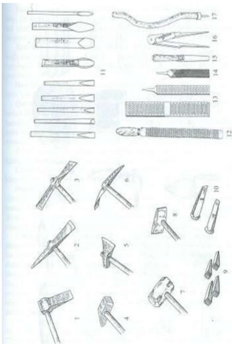
II tablo. Dərkəşmə və ölçməmə alətləri; 1,3 – Daş baltası; 2 – Döşən; 3 – Təvəz-tişək; 4 – Cökək; 6 – Qalaqburun; 7 – Güz; 8 – Tişək; 9 – Kiçik para; 10 – Böyük para; 11 – Düz və qırıqqa tişələr; 12,13 – Törpülər; 14 – Yarı yey; 15 – Mısq; 16 – Pəncə; 17 – Dənkaçan.
