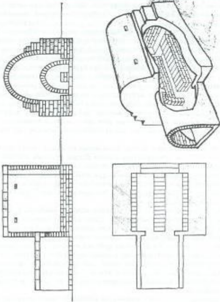
XIII tablo, K rpu l  dulus sobası. Lankaranın Səp zadı kandi.
