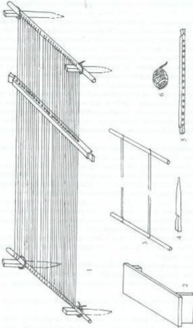
XXIX tablo. 1 - Hafir dazgahı; 2 - Oruracağ; 3 - Dazgahın dolğunları; 4 - Mıxca; 5 - Si (döyac); 6 - Ligatın yumuğı.
