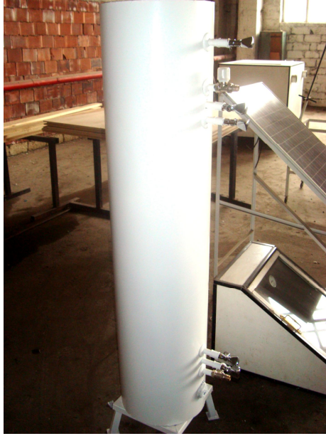
Şəkil 18.1. İkikonturlu istilikdəyişdiricinin ümumi görünüşü.
