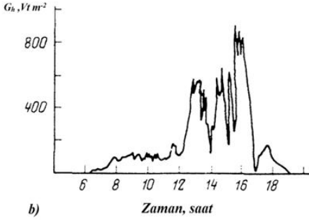
Şəkil 6.2. İlin müxtəlif fəsilərində üfüqi səthin şüalanması.
