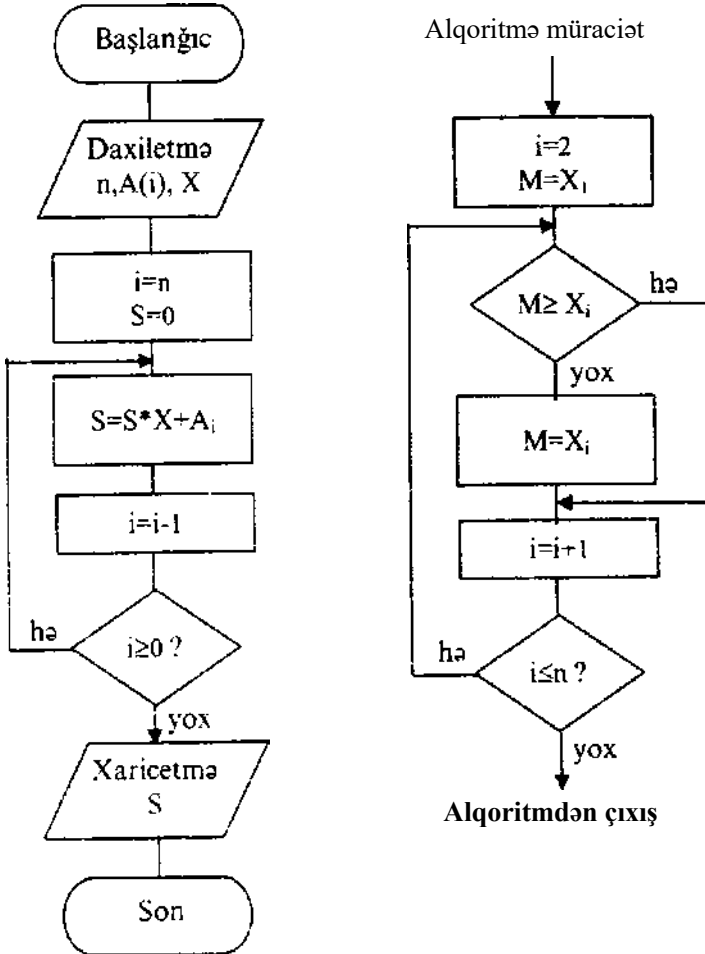
Şəkil 4.10. Hörner sxemi vasiləsilə Şəkil 4.11. X(n) massivinin ən böyük çoxhədlinin qiymətini hesablanması üçün elementlərin tapılması alqoritmi-alqoritminin təsviri
