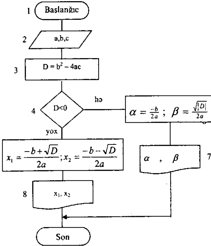
Şəkil 4.4. Kvadrat tənliyi üçün həll alqoritm
