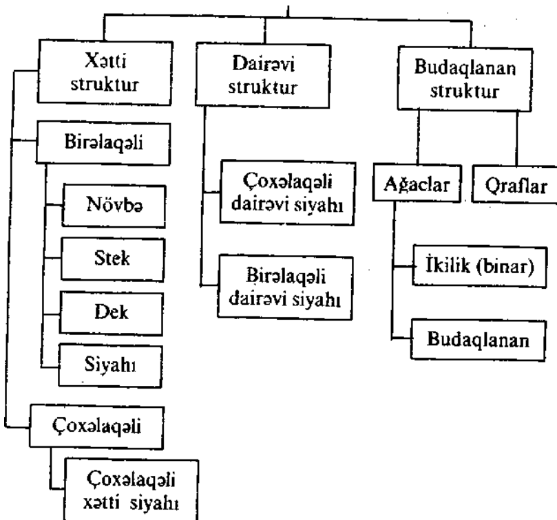
Şəkil 6.2. Əlaqəli dinamik verilənlərin növləri
