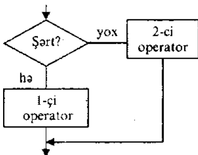
Şəkil 4.2. Tam formalı budaqlanma
