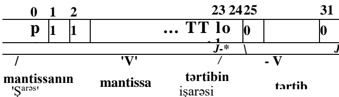
Şəkil 2.4. Sürüşən nöqtəli ədədlərin kompüterdə təsviri
