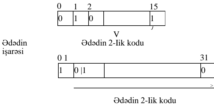
Şəkil 2.3. Tam və sabit nöqtəli ədədlərin kompüterdə təsviri
