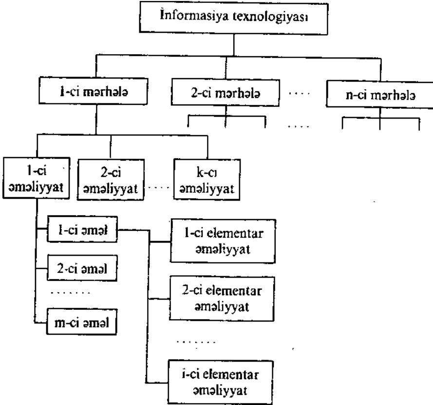
Şəkil 1.4. İnformasiya texnologiyasının iyerarxik struktur şəklində təsviri
