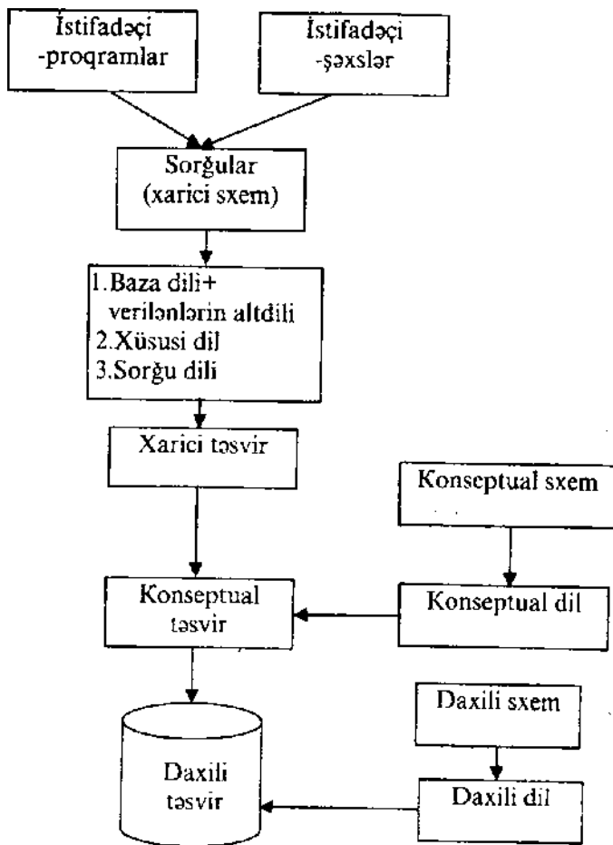
Şəkil 12.11. Verilənlərin təsvir səviyyələri və dilləri arasında əlaqə Hər istifadəçinin özünün
