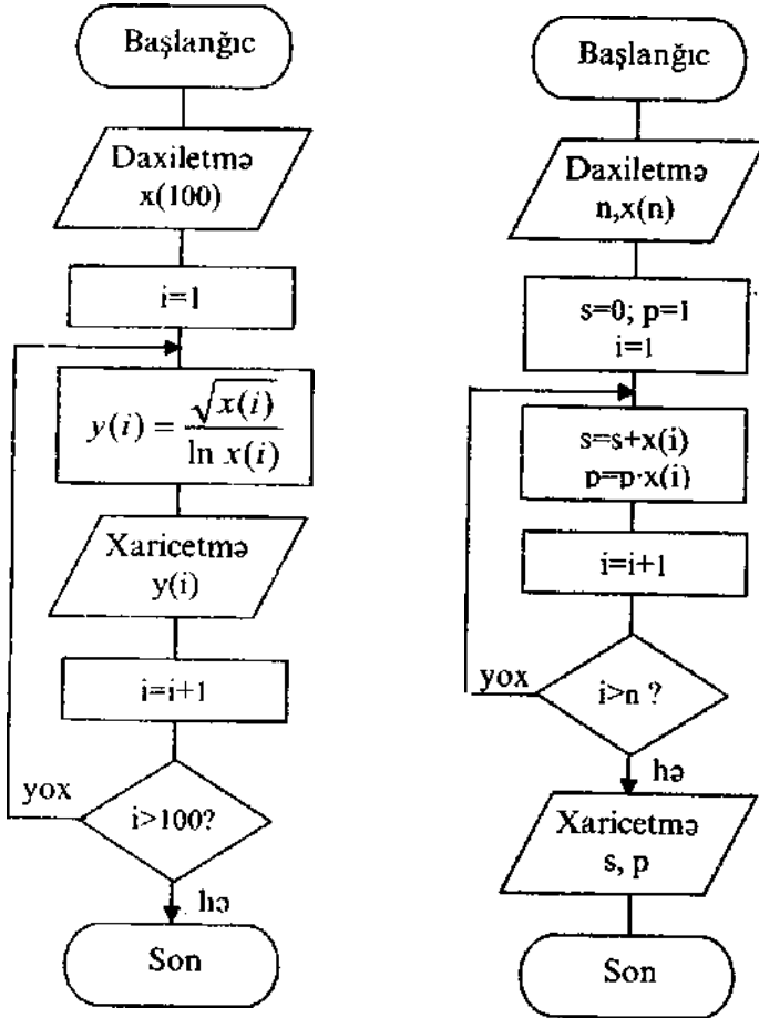
Şəkil 4.8. Arqumentin qiymətlər çoxluğu - Şəkil 4.9. Massivin elementləri - gına görə funksiyanın qiymətlər çoxluğu - nin cəminin və hasilini hesablayan qunu hesablayan alqoritmin blok-sxemi alqoritmin blok-sxemi
