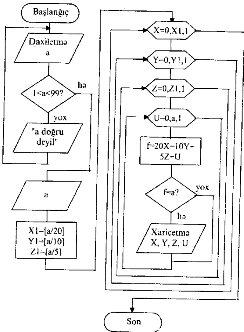
Şah! 4.14. Misal 12-nin həllini təmin edən algoritmin blok-sxemi
