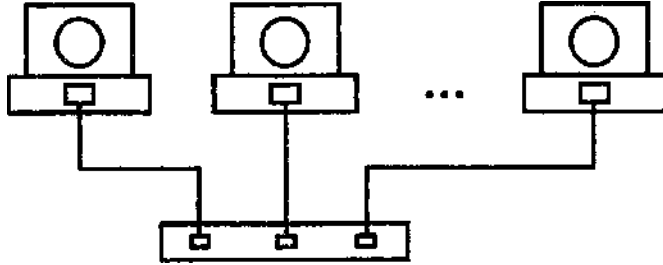
Şəkil 15.1. "Ulduz" topologiyası
