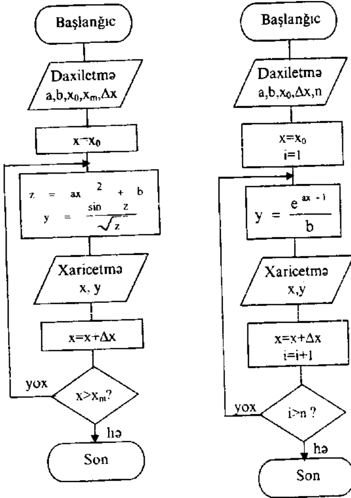
Səkil 4.6. Dövrələr sayı veril- Şəkil 4.7. Dövrələr sayı verilən məyən monoton dəyişənli hesab- monoton dəyişənli hesablama lama
