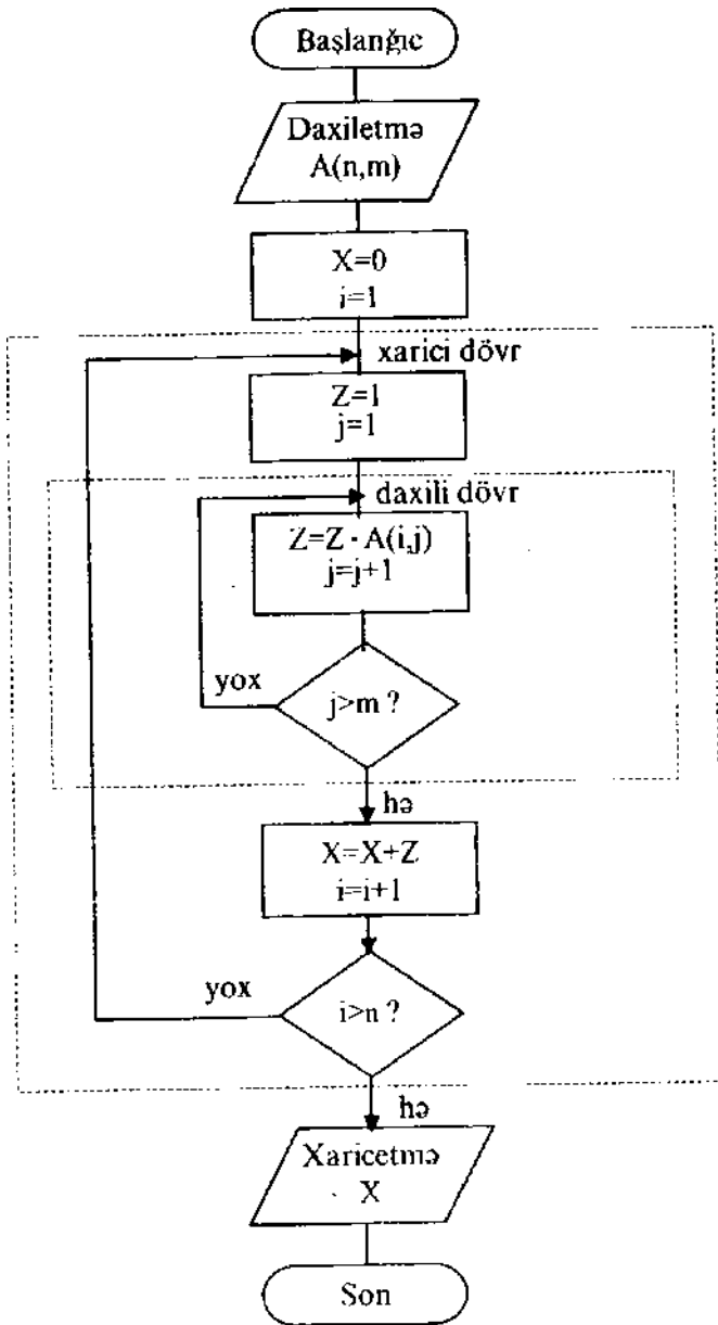
Şəkil 4.12. Mürəkkəb dö'm algoritma aid misal
